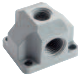
Type VDK-138, voorzien van 3/8" boven & 1/2" voor. BSP female
