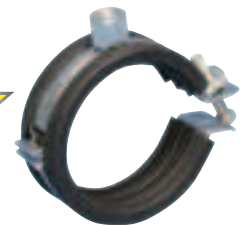
Super fix - light - enkel - gegalvaniseerde scharnierende pijpbeugel, epdm inlage, M8, voor snelmontage 12-61 mm
